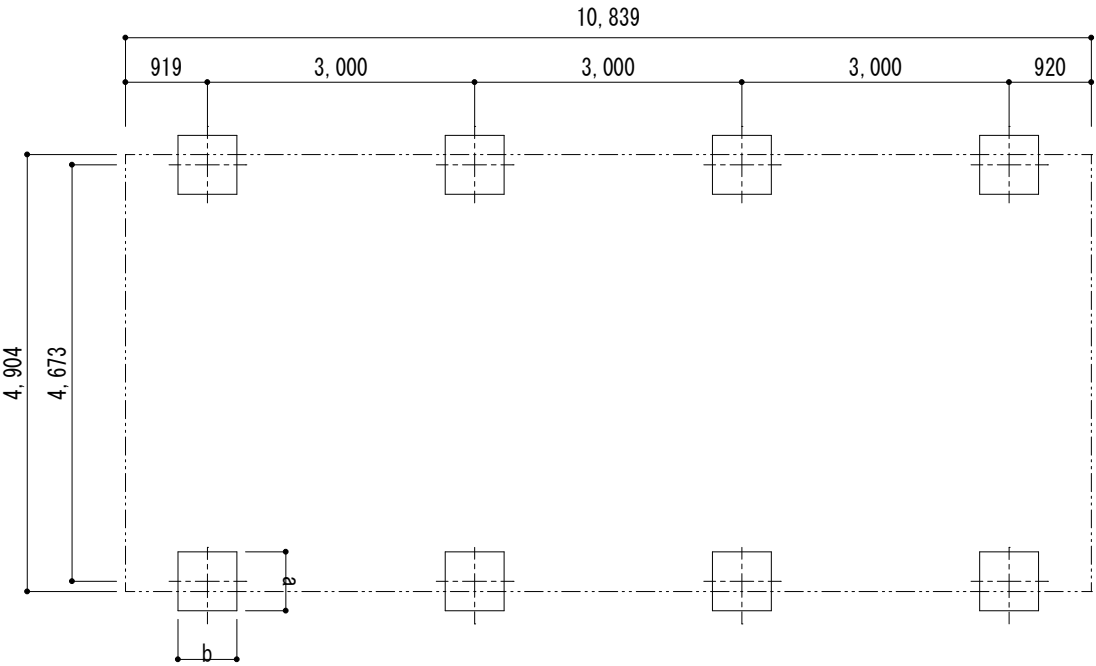
■基礎配置図
